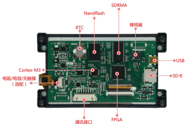
图 1-4 硬件配置图
